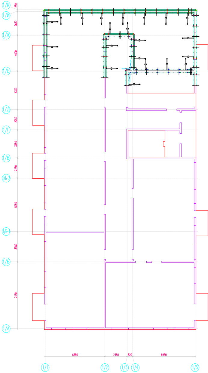
Захватка №1
