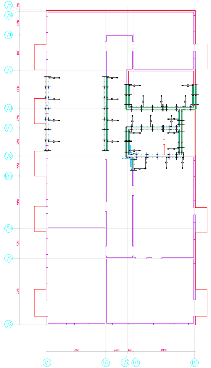
Захватка №2
